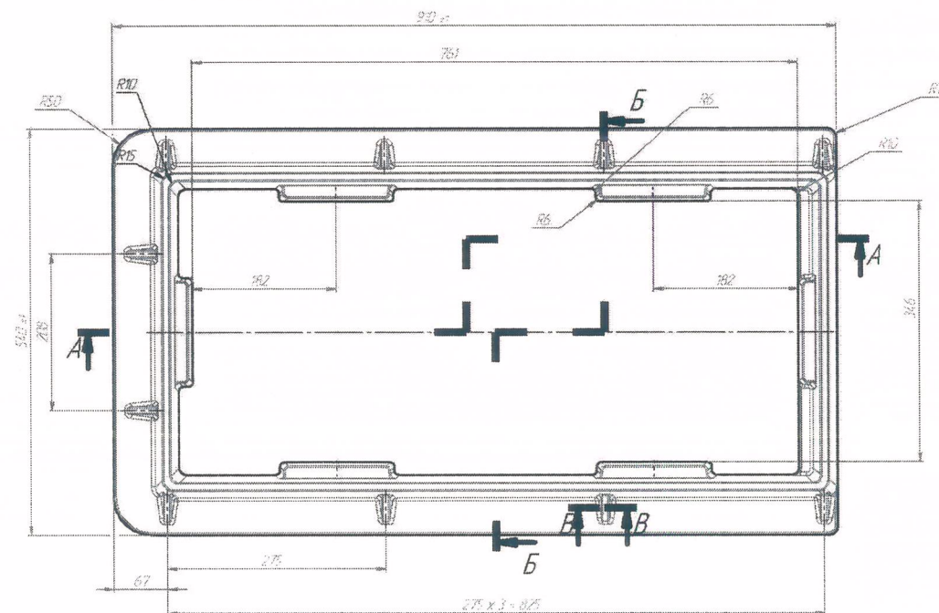
Люк чугунный прямоугольного дождеприемника тип «ДБ1» (В125) 1 - 78 * 36 ГОСТ 3634-2019 (торцевое прилегание)
